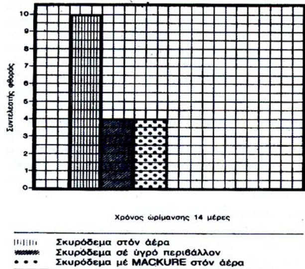
Σχ. 2: Δοκιμή αντοχής σε φθορά σε δοκίμια 190x190x38 mm
