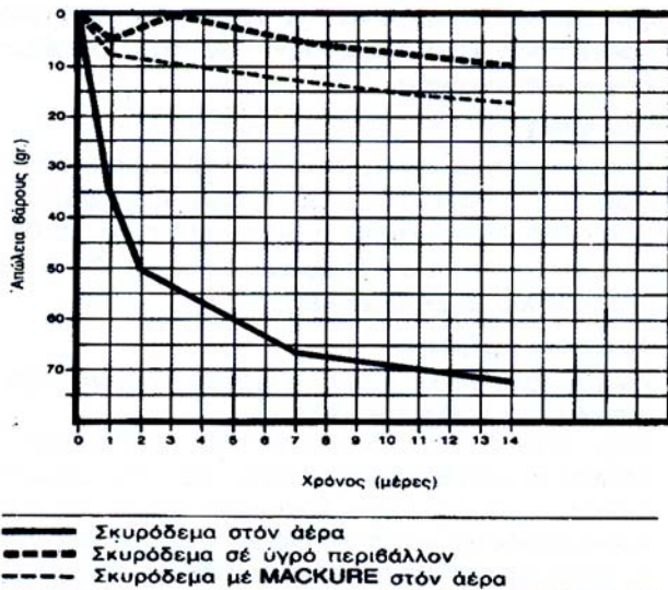
Σχ. 1: Απώλεια θάρους ελεγχόμενη σε δοκίμια 190x190x38 mm
